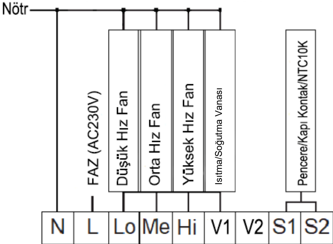
2 Borulu Sistem Bağlantısı
