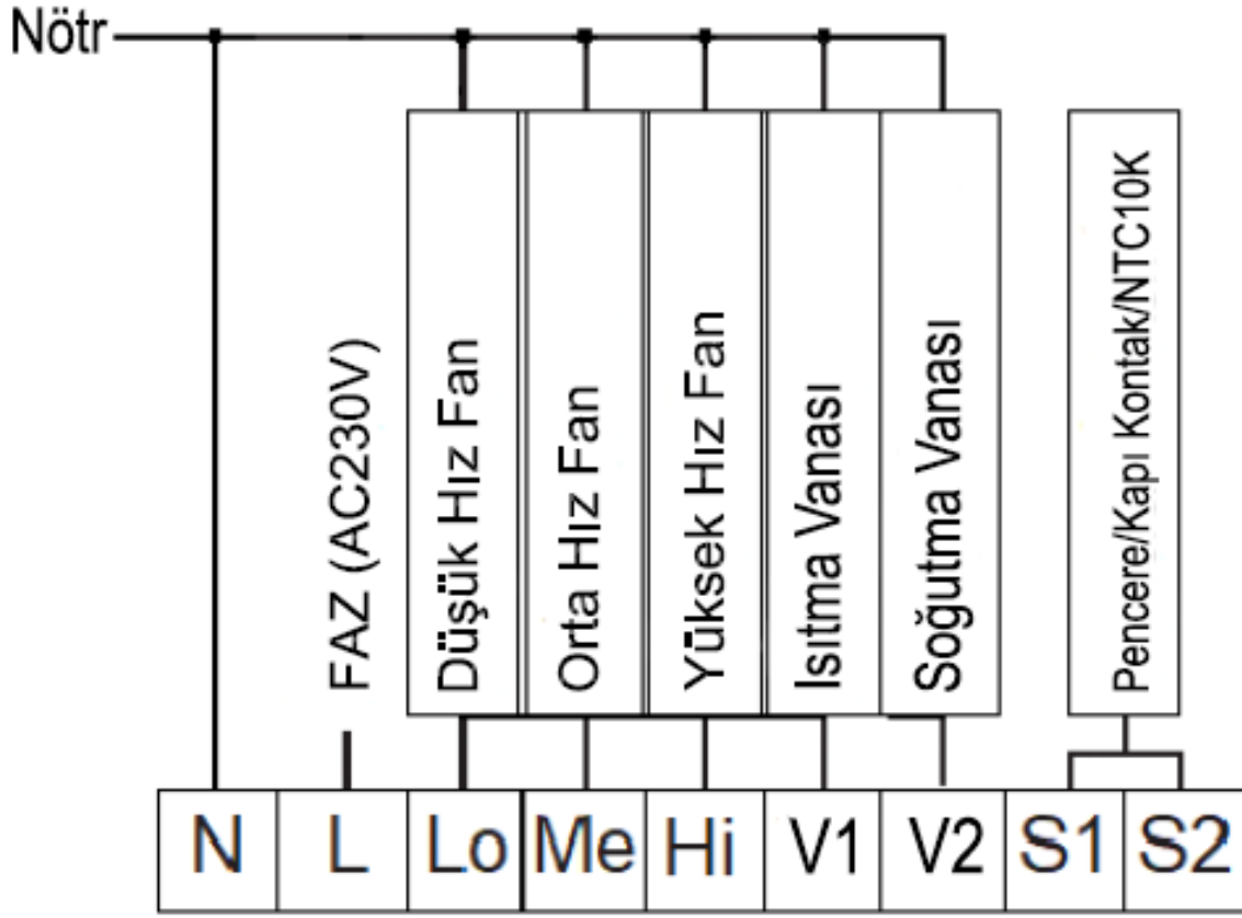
4 Borulu Sistem Bağlantısı
